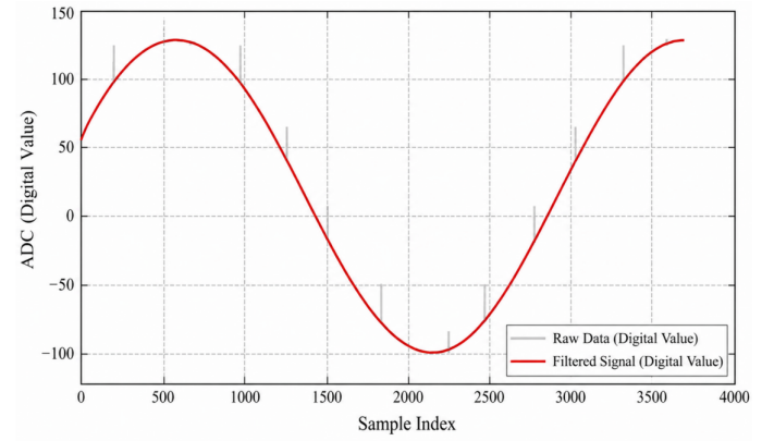
a) 32kHz/250mVpp
