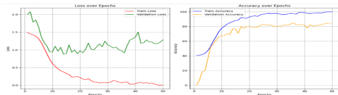
Figure 7. ViT.
