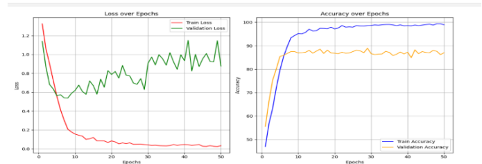
Figure 9. EfficientNet-B0 + ViT.
