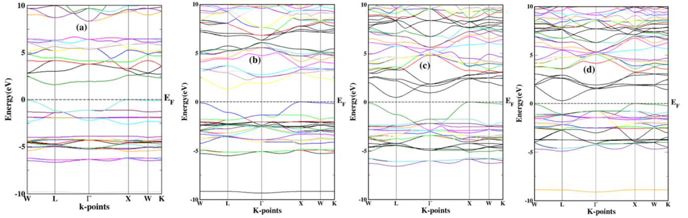
Figure 1. Band structures of (a) \text{Li}_2\text{AgSbF}_6 , (b) \text{Li}_2\text{AgSbCl}_6 , (c) \text{Li}_2\text{AgSbBr}_6 , and (d) \text{Li}_2\text{AgSbI}_6 .
