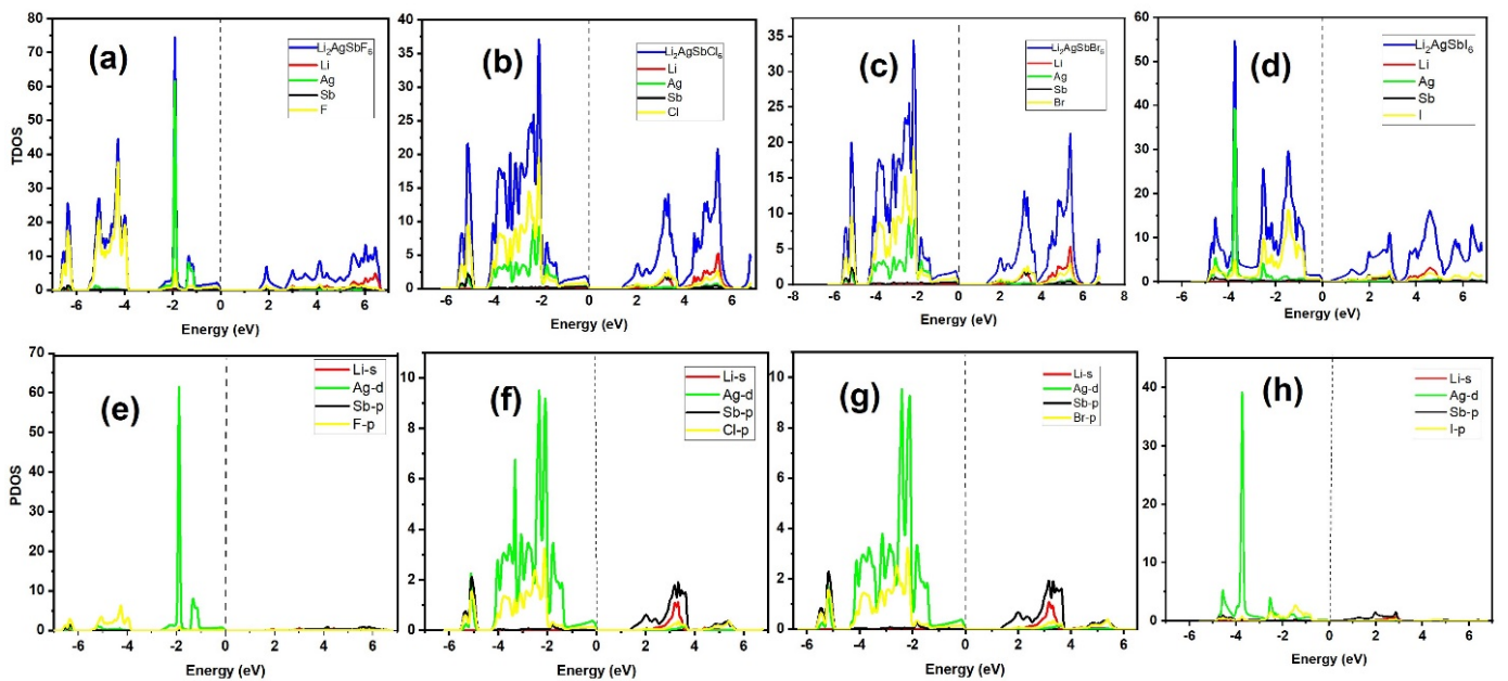
Figure 2. TDOS of (a) \text{Li}_2\text{AgSbF}_6 , (b) \text{Li}_2\text{AgSbCl}_6 , (c) \text{Li}_2\text{AgSbBr}_6 , and (d) \text{Li}_2\text{AgSbI}_6 , and PDOS of (e) \text{Li}_2\text{AgSbF}_6 , (f) \text{Li}_2\text{AgSbCl}_6 , (g) \text{Li}_2\text{AgSbBr}_6 , and (h) \text{Li}_2\text{AgSbI}_6 .
