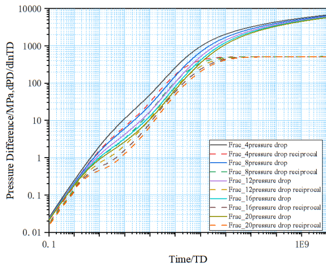
(a) k=0.05\text{md}
